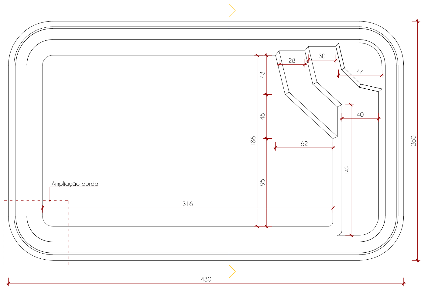
Vista superior
