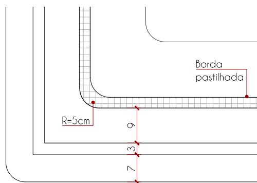
Ampliação borda 1/10
