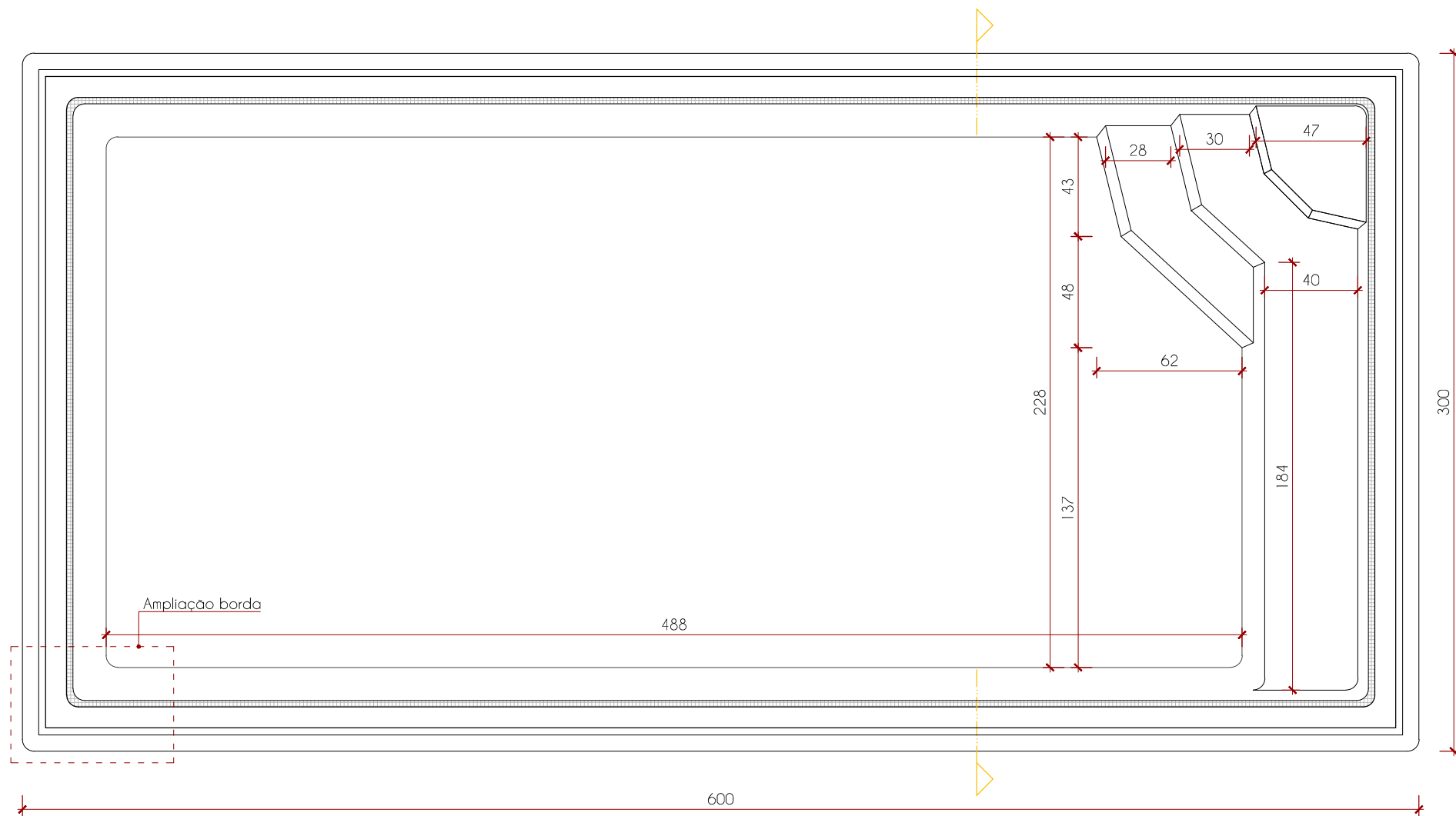
Vista superior
