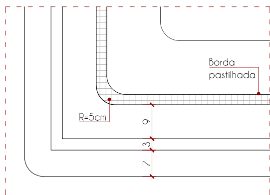
Ampliação borda 1/10
