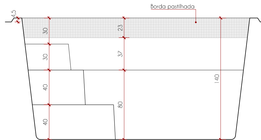
Corte
