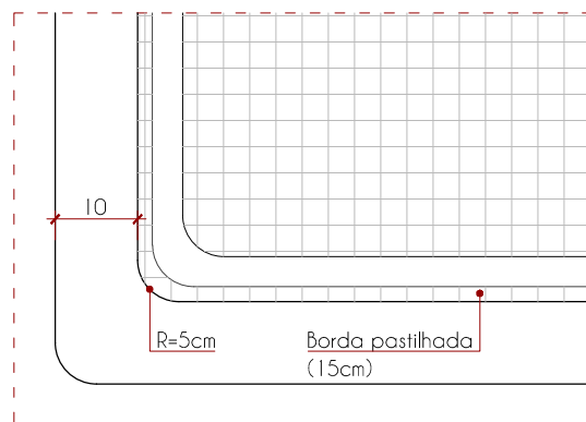
Ampliação borda 1/10
